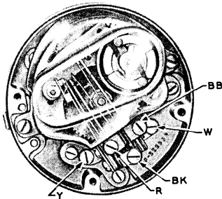
FIG. 4—6A DIAL
